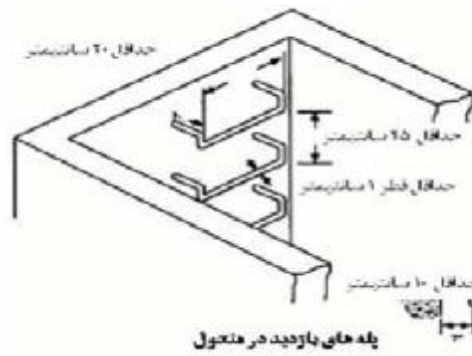
شکل ۲۲- پلکان متعول
