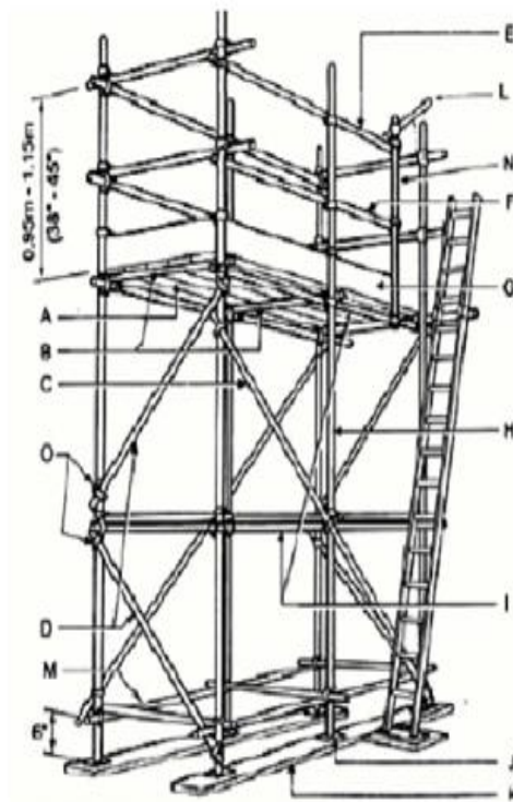
شکل ۴۶- داربست با کلیه اجزاء
