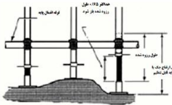
شکل ۵۱ - نحوه برپایی داربست
