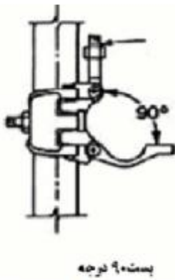
شکل ۴۰- بست ۹۰ درجه
