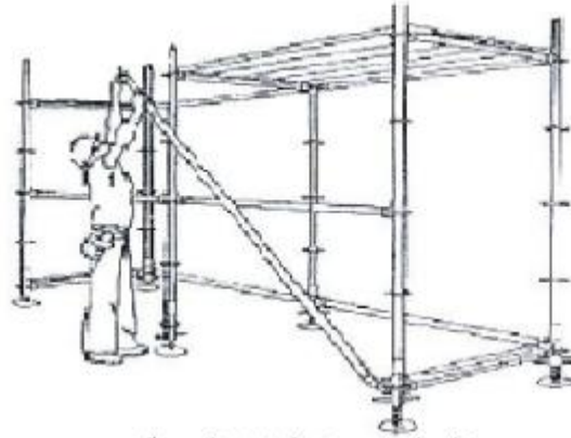
شکل ۵۰ - نحوه بستن یادبند در داربست ثابت
