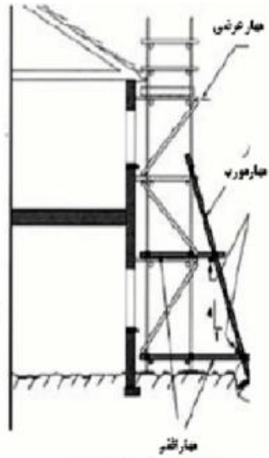
شکل ۴۲- مهار مورب داربست
