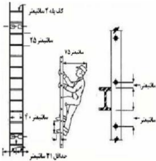
شکل ۱۸- نحوه بالا رفتن از نردبان ثابت با محفظه حمل‌وی
