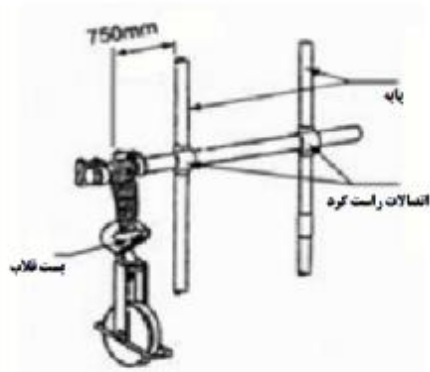
شکل ۴۱- بست اتصال فرقره
