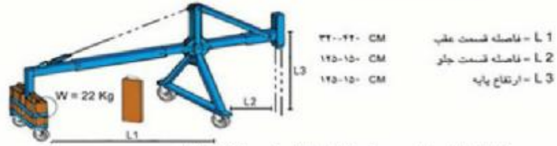
شکل ۱۲۰- ابزار برای نصب روی بام با بالاترین ارتفاع سازه در جایگاه کار آویزان
